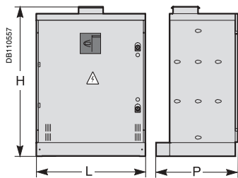
Armoire A2 sans disjoncteur de tête.
