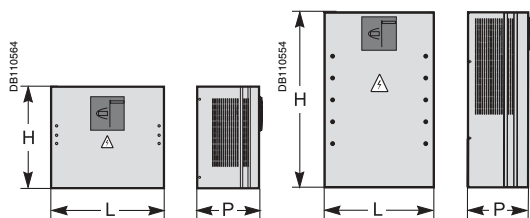
Coffret C1 sans disj. de tête. Coffret C2 sans disj. de tête.
