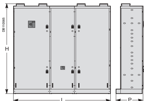
Armoire A4B avec disjoncteur de tête.
