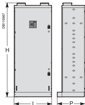
Armoire A3 sans disjoncteur de tête.
