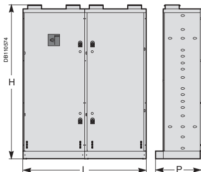
Armoire A4 sans disjoncteur de tête.
