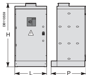
Armoires A1 et A2 sans disj. de tête.
