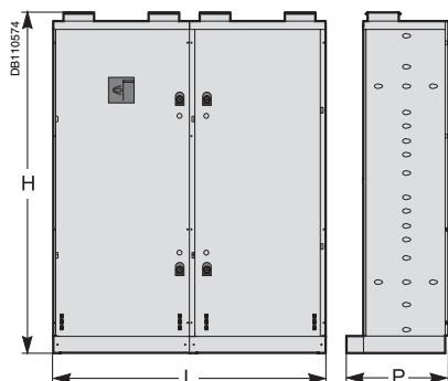
Armoire A4 sans disj. de tête.
