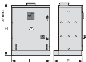
Armoire A2 avec disj. de tête.
