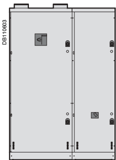
Armoire A3B avec disjoncteur de tête.
