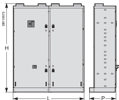
Armoire A4 avec disj. de tête.
