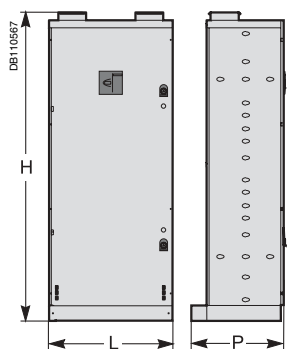
Armoire A3 sans disj. de tête.
