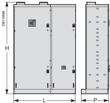
Armoire A3B avec disjoncteur de tête.
