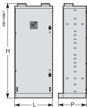
Armoire A3 sans disjoncteur de tête.
