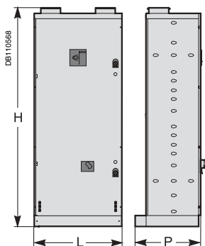
Armoire A3 avec disj. de tête.
